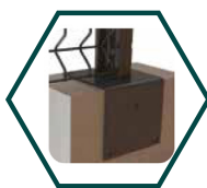
Platine équerre 200x200mm : panneau jusqu'à 2m05. Nécessite vis M8x16 (non fournies).
